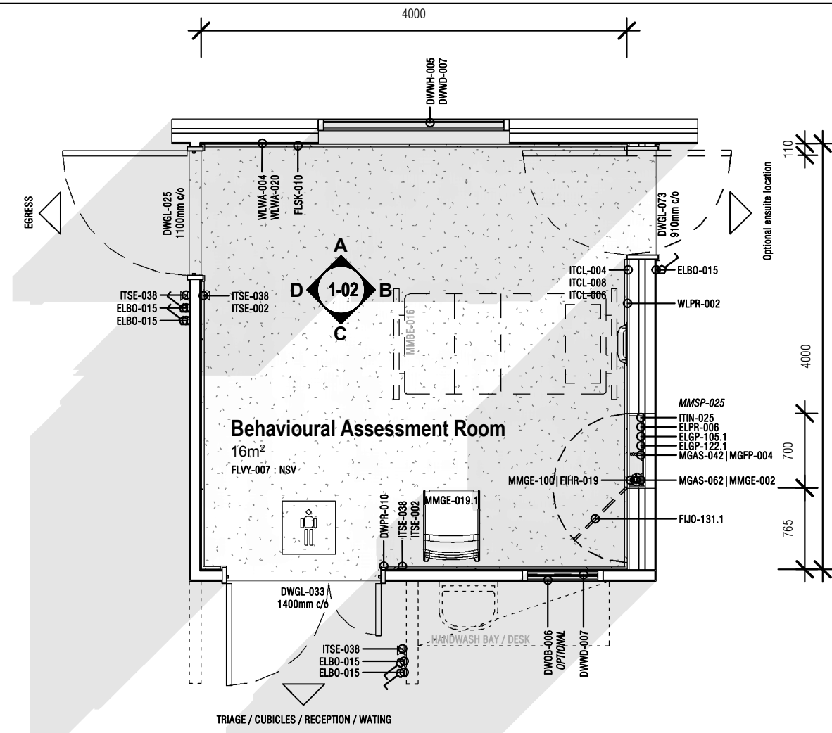
② PLAN - BAR 16m2 1 : 50
