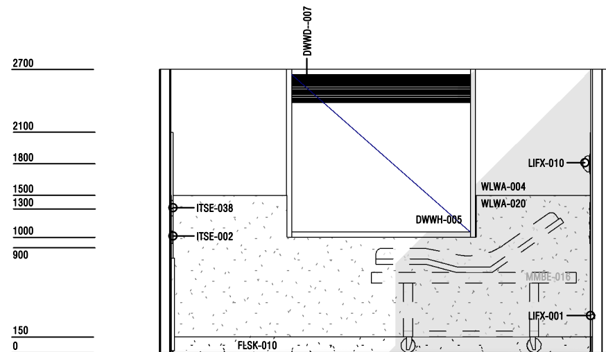
A ELEVATION - BAR 1 : 50
