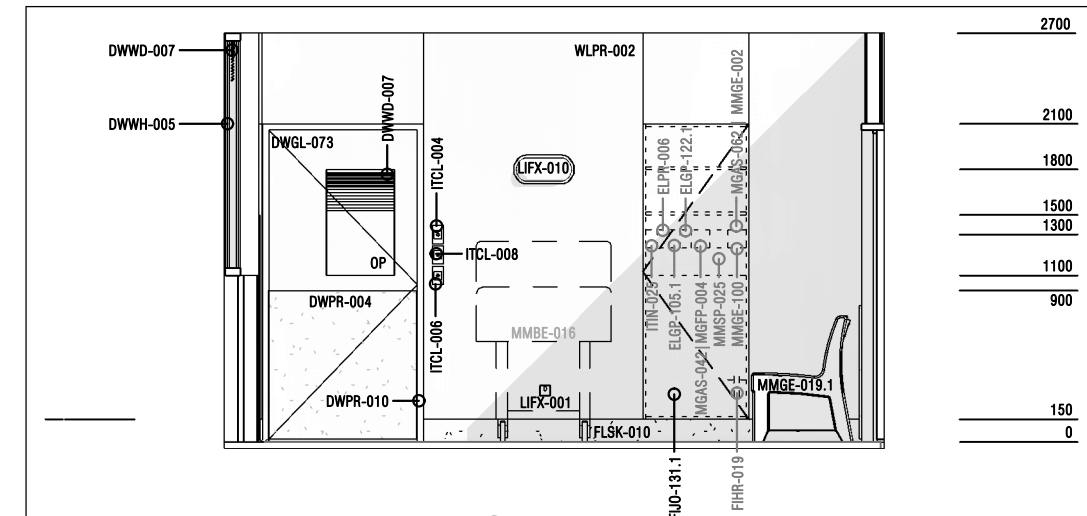
B ELEVATION - BAR 1 : 50
