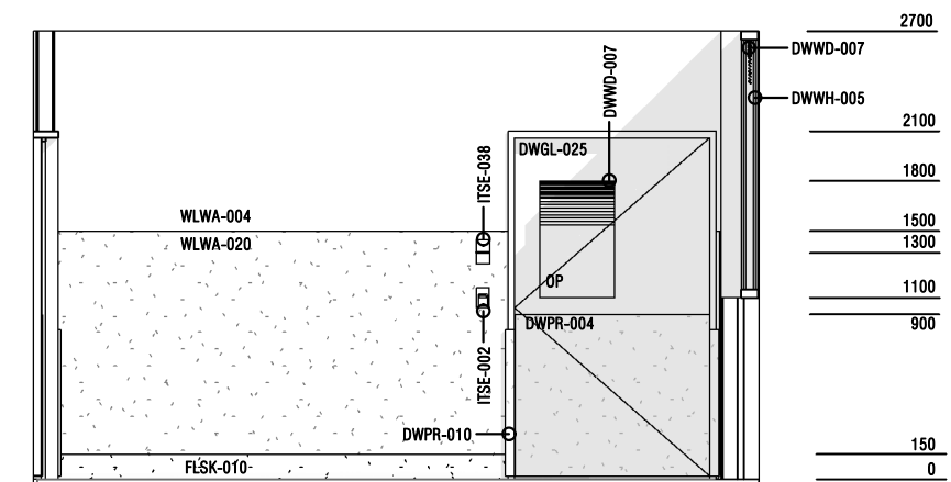
D ELEVATION - BAR 1 : 50
