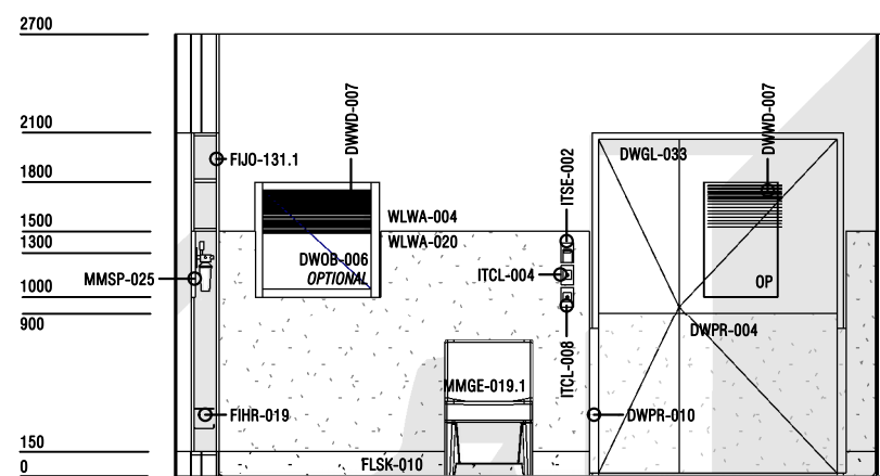
C ELEVATION - BAR 1 : 50
